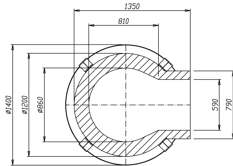
SEZIONE IN PIANTA INTERNO FORNO
